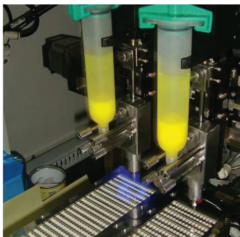
Люминофор из шприцов заливается в корпуса
